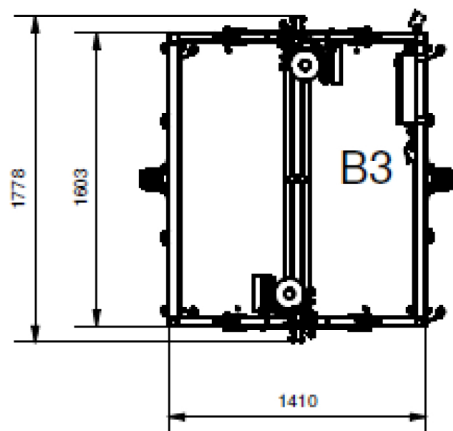
Configuration 8 Plate-forme 1600x1410 0654210007
